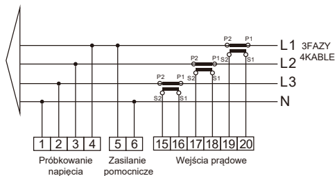
Rys. 7.3 Licznik Eastron
