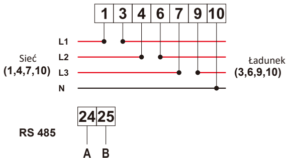
Rys. 7.5 Licznik CHNT
