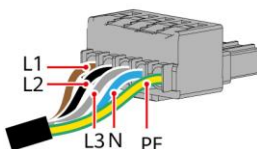
Zaciski po stronie falownika (trójfazowego)
